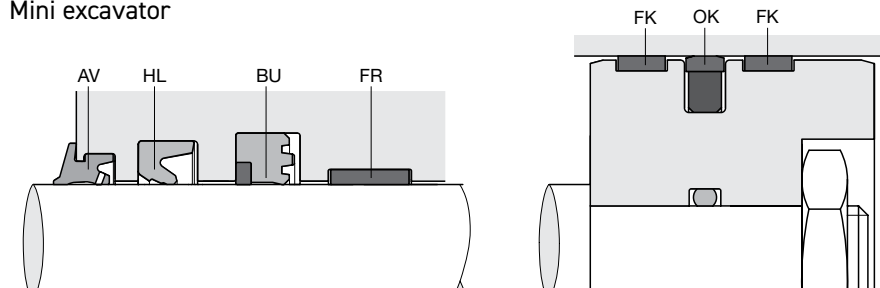
Mini excavator
