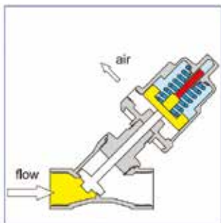
常闭阀门
