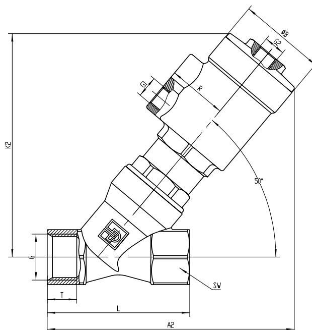
常开阀
