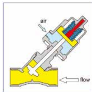
常开阀门
