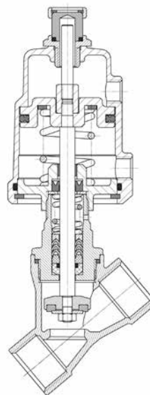
常开阀门
