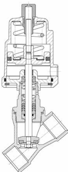
常闭阀门
